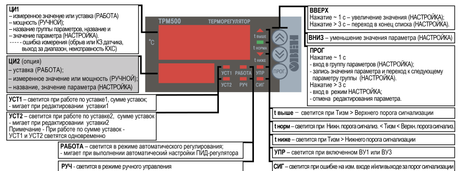
Рисунок 5 – Назначение ЦИ, кнопок и светодиодов
