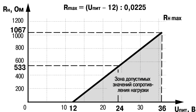
Рисунок 5.7 – График для выбора допустимых значений сопротивления нагрузки
