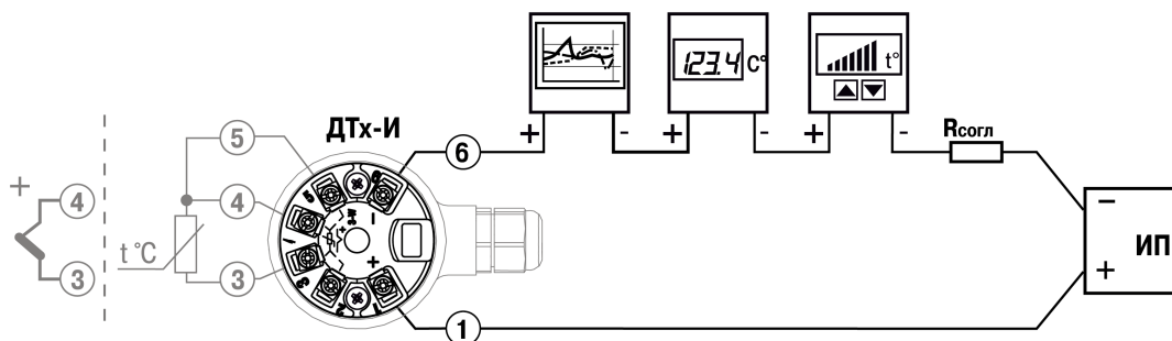
Рисунок 5.8 – Схема подключения датчика к нескольким вторичным приборам
