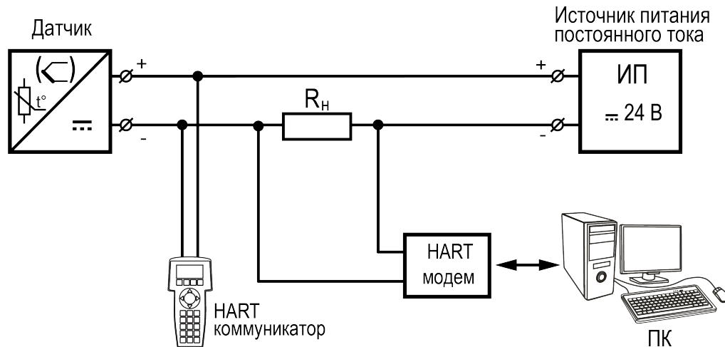
Рисунок 5.9 – Подключение датчиков ДТх-И[Н] к ПК
