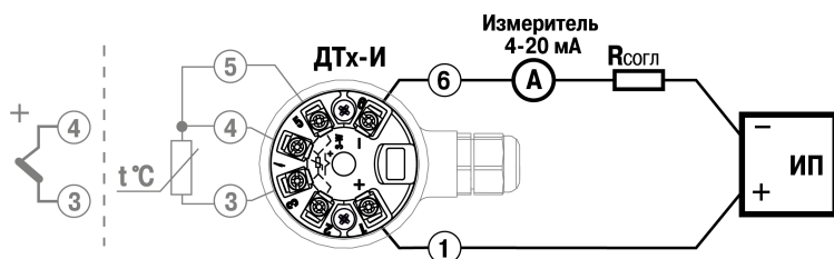
Рисунок 5.5 – Схема подключения
