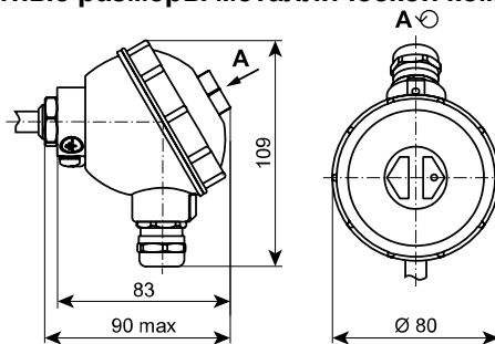
Рисунок Г.3 – Габаритный чертеж металлической коммутационной головки ДТС305М, ДТС505М, ДТС515М
