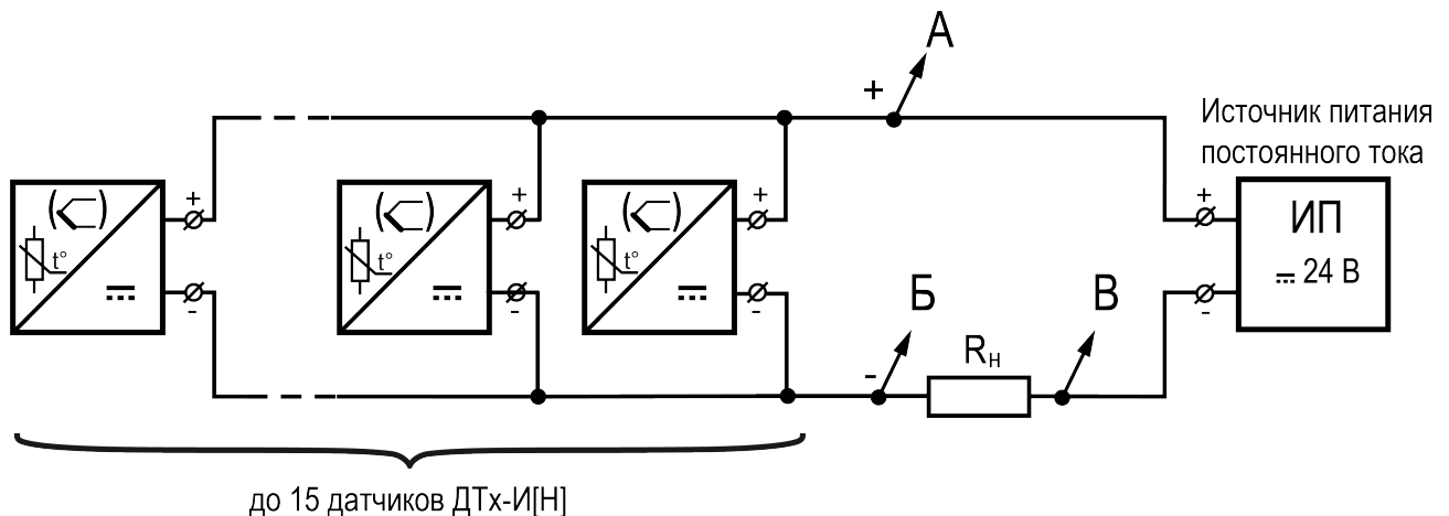
Рисунок 5.10 – Пример системы с параллельным подключением датчиков
