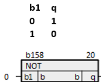
Рисунок 10.33 – Логическое НЕ (NOT)
