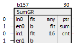
Рисунок 10.24 – Сложение некоторых слагаемых (SumGR)
