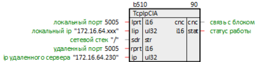
Рисунок 10.157 – TCP/IP клиент (TcpIpCIA)
