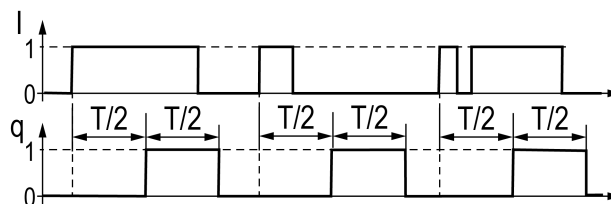
Рисунок 10.69 – Алгоритм блока HalfPulse
