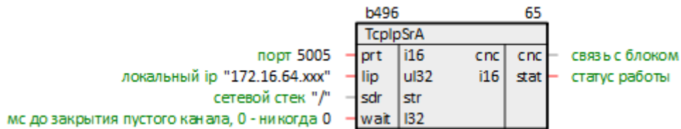
Рисунок 10.158 – TCP/IP сервер (TcpIpSrA)
