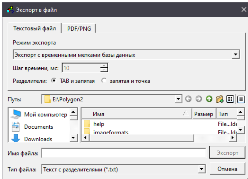
Рисунок 3.23 – Экспорт графика
