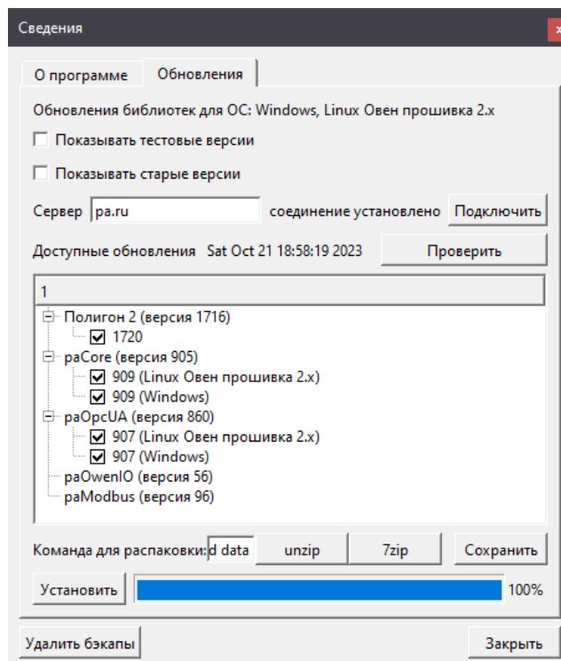
Рисунок 1.31 – Окно Обновления
