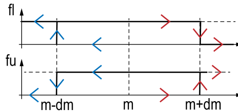
Рисунок 10.134 – Алгоритм SmTrig
