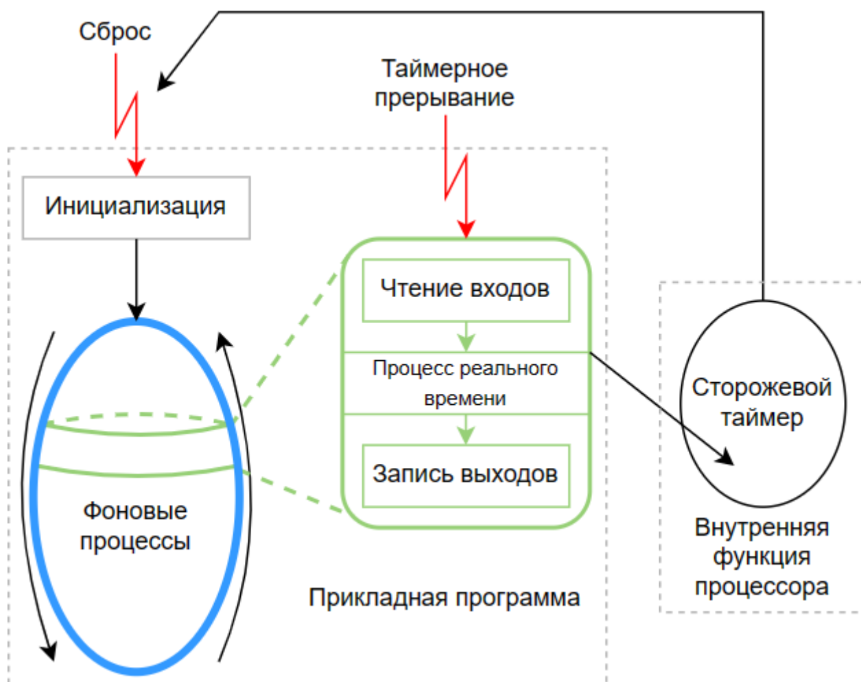
Рисунок 2.3 – Поток данных
