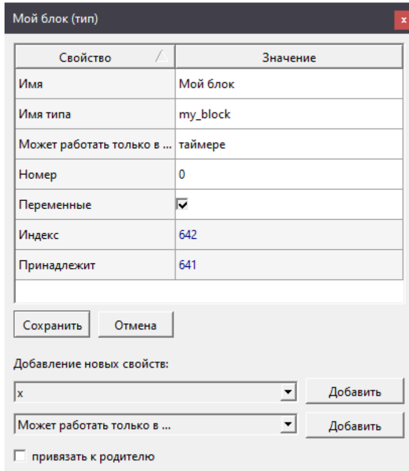
Рисунок 8.48 – Свойства Типа
