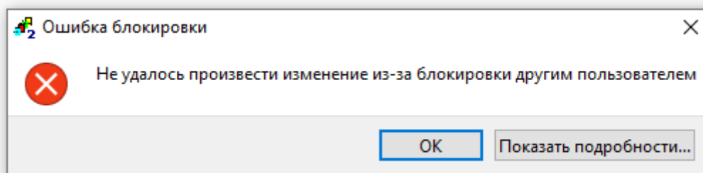
Рисунок 8.83 – Ошибка блокировки
