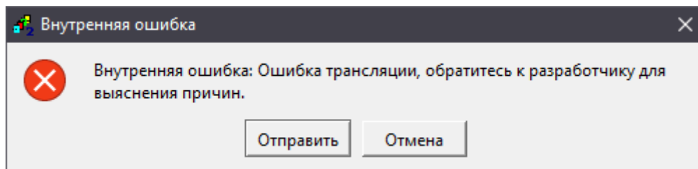
Рисунок 1.40 – Ошибка трансляции
