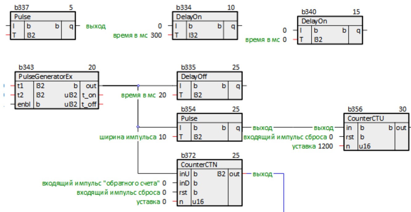
Рисунок 4.43 – Порядок выполнения по потоку данных
