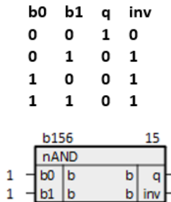
Рисунок 10.32 – Логическое НЕ-И (nAND)
