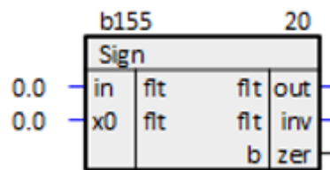
Рисунок 10.28 – Определение знака (Sign)
