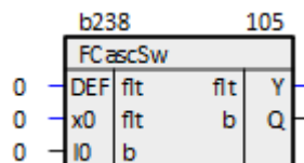
Рисунок 10.60 – Выбор одного из вещественных значений (FCascSw)
