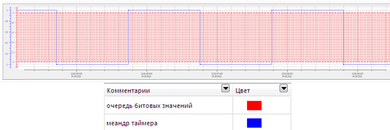
Рисунок 10.171 – Очередь битов qb
