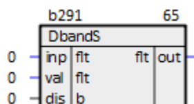
Рисунок 10.98 – Симметричная мертвая зона (DbandS)
