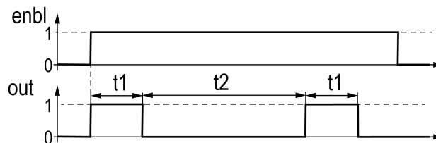
Рисунок 10.76 – Алгоритм блока PulseGeneratorEx
