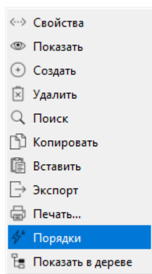
Рисунок 4.39 – Порядки
