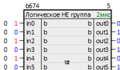
Рисунок 8.47 – Работа блока
