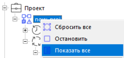
Рисунок 1.38 – Показать все
