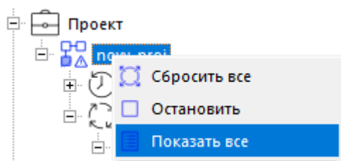
Рисунок 7.14 – Показать все
