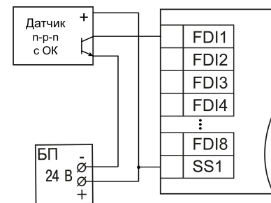
Рисунок 13 – Подключение транзисторов типа п-р-п
