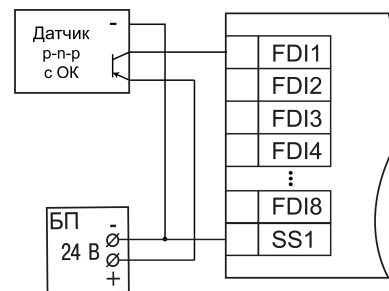
Рисунок 12 – Подключение транзисторов типа р-п-р
