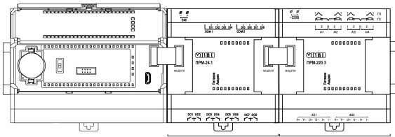
Рисунок 14 – Расположение модулей расширения на шине
