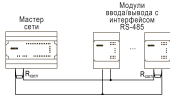
Рисунок 13 – Типовая схема подключения в режиме Master
