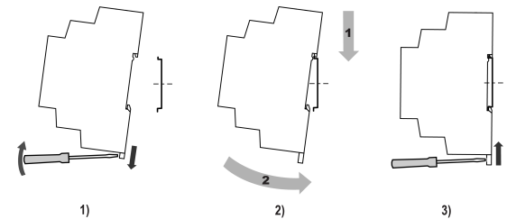
Рисунок 1 – Монтаж прибора
