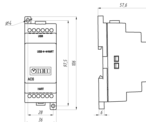
Рисунок 1 – Габаритные размеры
