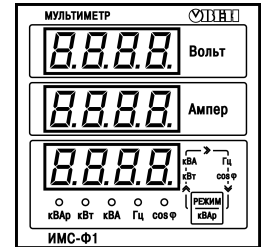
Рисунок 6.2 – Лицевая панель
