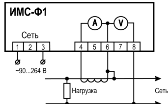
Рисунок 5.3 – Схема подключения с трансформатором
