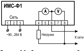
Рисунок 5.2 – Схема подключения без трансформатора
